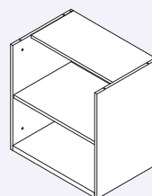
Módulo sin led. Ancho 60,8 cm / Alto 64 cm
