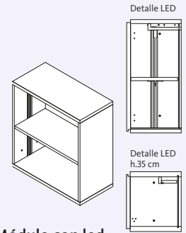
Módulo con led. Ancho 60,8 cm / Alto 67 cm
