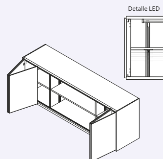
Módulo con led. Ancho 184,4 cm / Alto 67 cm
