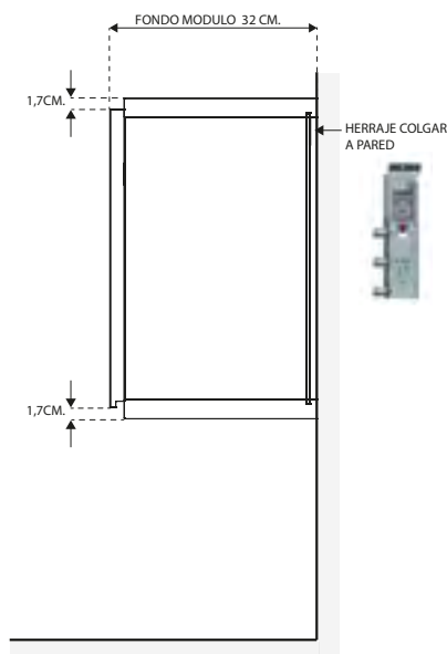
Módulo No apilable para colgar
