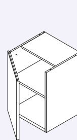
Módulo sin led. Ancho 60,8 cm / Alto 64 cm
