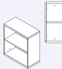
Módulo sin led. Ancho 60,8 cm / Alto 67 cm
