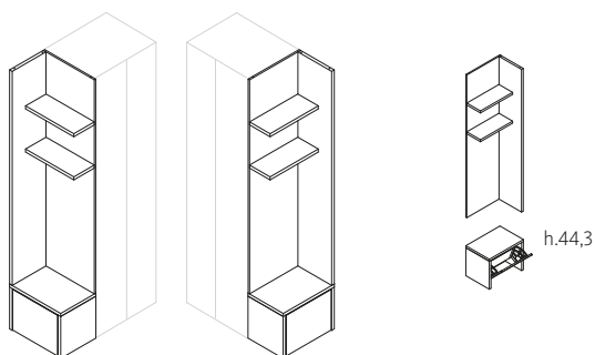
① Terminal banco zapatero Izq. / Dch.
