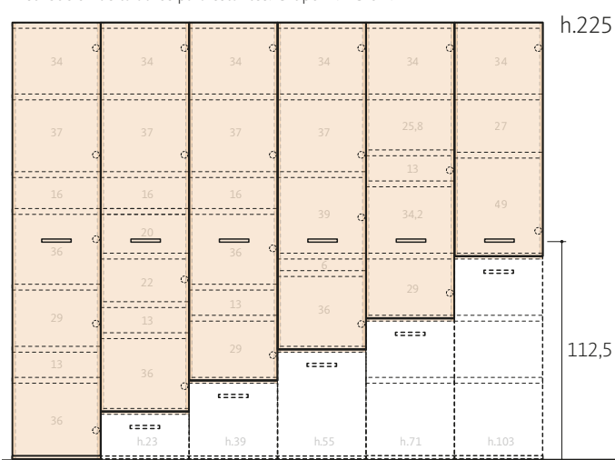
Distribución de taladros para estantes. Grupo h.225 cm.
