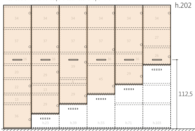
Distribución de taladros para estantes. Grupo h.202 cm.
