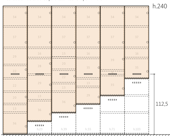
Distribución de taladros para estantes. Grupo h.240 cm.
