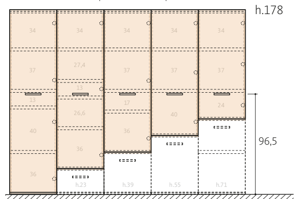
Distribución de taladros para estantes. Grupo h.178 cm.
