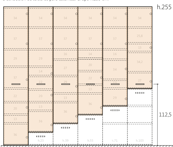
Distribución de taladros para estantes. Grupo h.255 cm.
