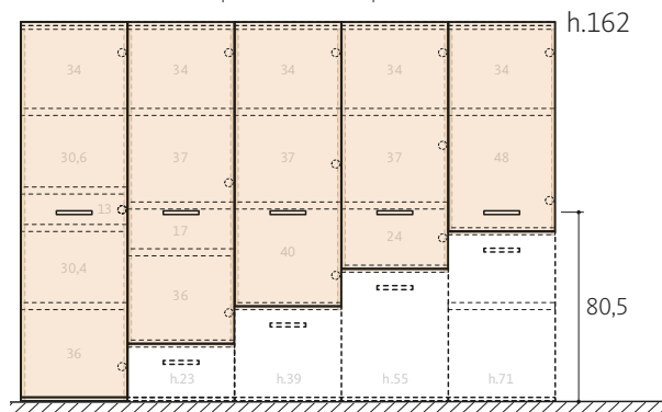
Distribución de taladros para estantes. Grupo h.162 cm.
