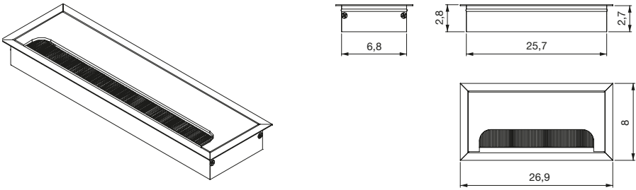
Pasacables metálico con tapa
