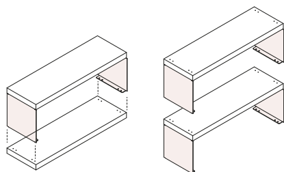
Módulo base: 1 ud.
