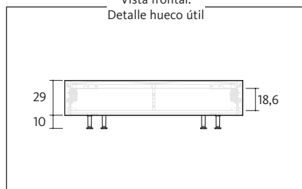
Vista frontal: Detalle hueco útil
