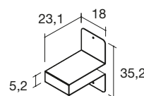
escuadra para estantes de grueso 5
